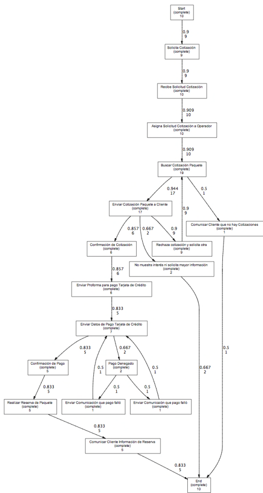
Figura 10. Modelo de proceso descubierto por el Heuristic Miner Fuente: elaboración propia.
