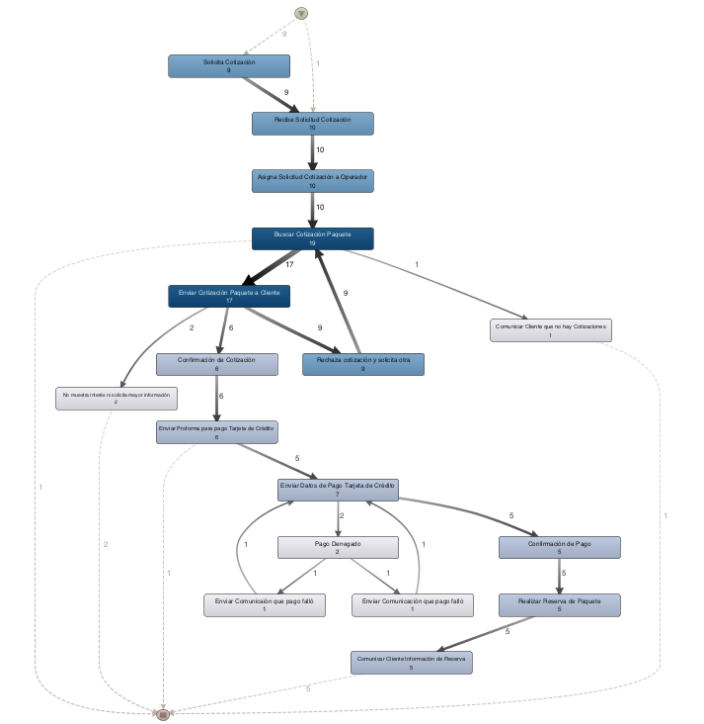
Figura 8. Modelo del proceso Fuente: elaboración propia.
