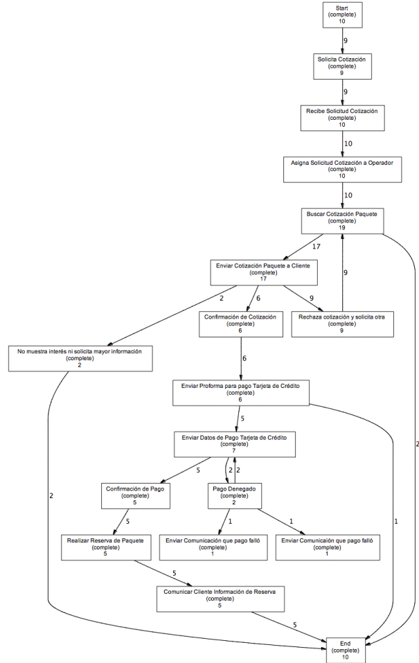
Figura 11. Modelo de proceso descubierto por el Genetic Miner Fuente: elaboración propia.
